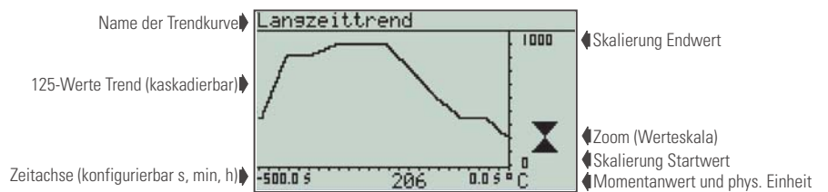
Fig. 7 Trendanzeige (VTREND)
